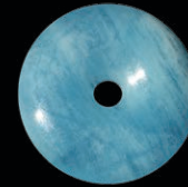
Aquamarin von der Fundstelle, die schon in der Antike wichtig war: 6.5 cm grosse Kugel und 4.5 cm grosse Pi-Scheibe aus Tamil Nadu, Indien.
